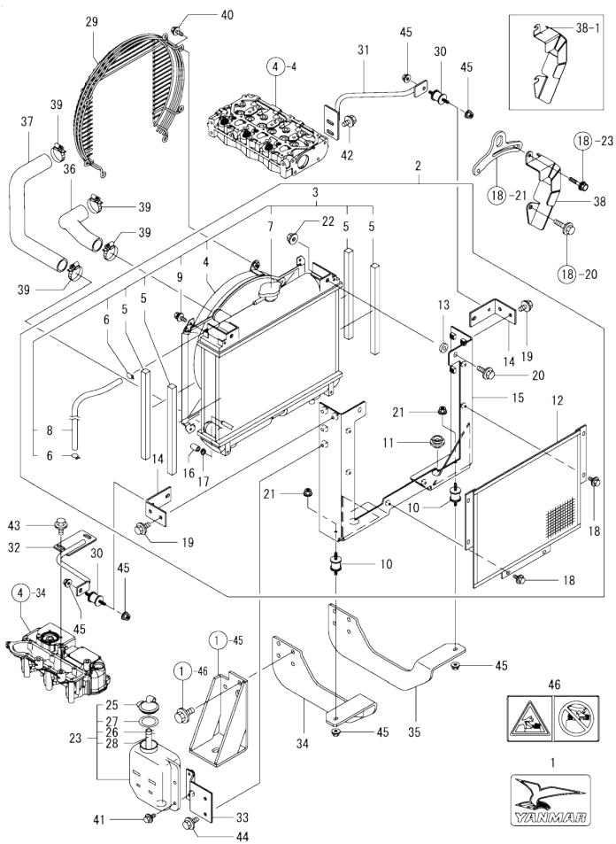
Fig.11. RADIATOR
